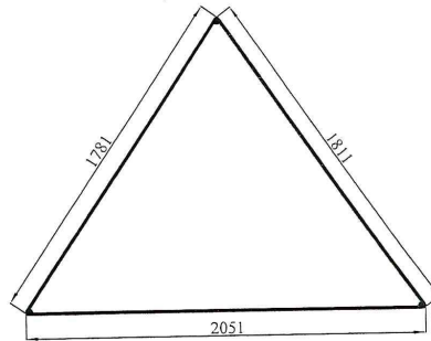
SEGMENT br. 3A (kom. 5)
