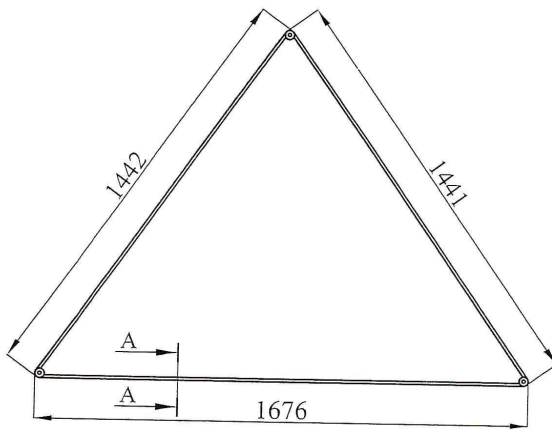
SEGMENT br. 1 (kom. 30)
